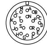
MS3102A20-29P Encoder Cable Connector 접속도
