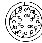
MS3102A20-29P Encoder Cable Connector 접속도
