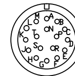
MS3102A20-29P Encoder Cable
